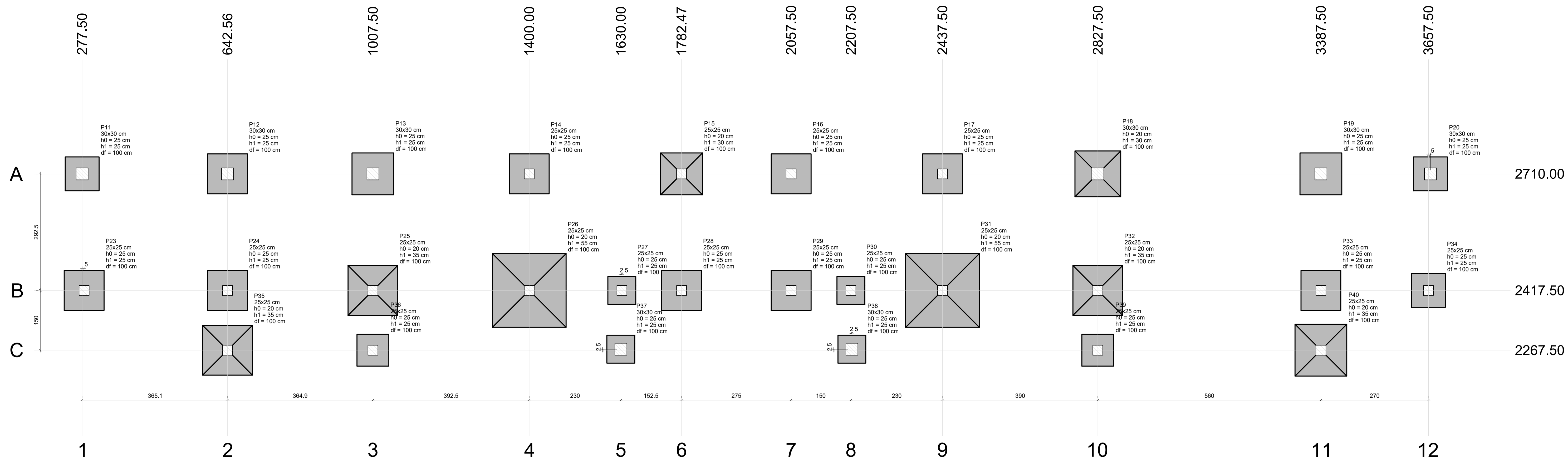
Planta de localização escala 1:50
