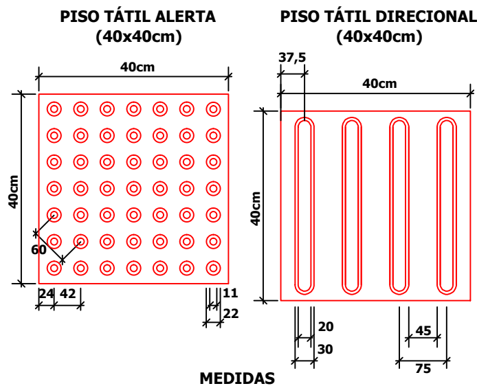
PISO TÁTIL / ACESSO À PROPRIEDADES PARTICULARES
