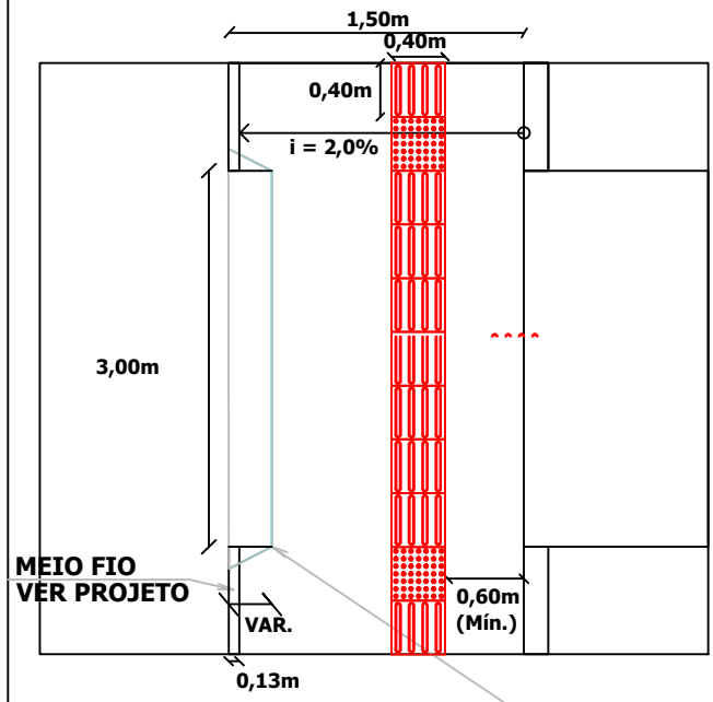
PISO TÁTIL / ACESSO À PROPRIEDADES PARTICULARES
