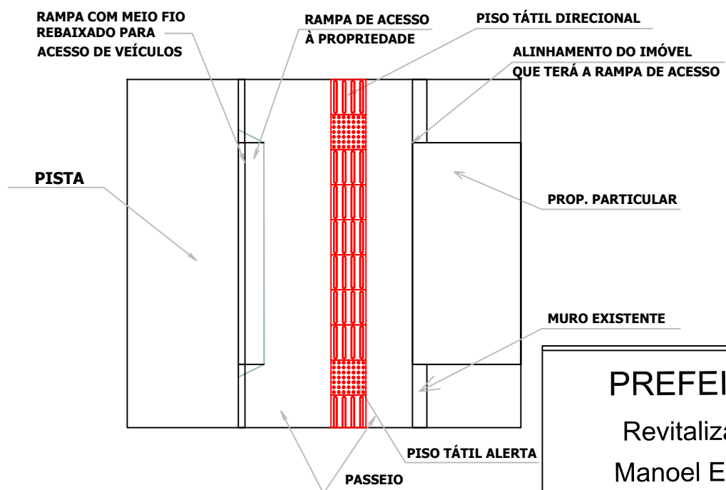
VISTA SUPERIOR PISO TÁTIL / ACESSO À PROPRIEDADES PARTICULARES
