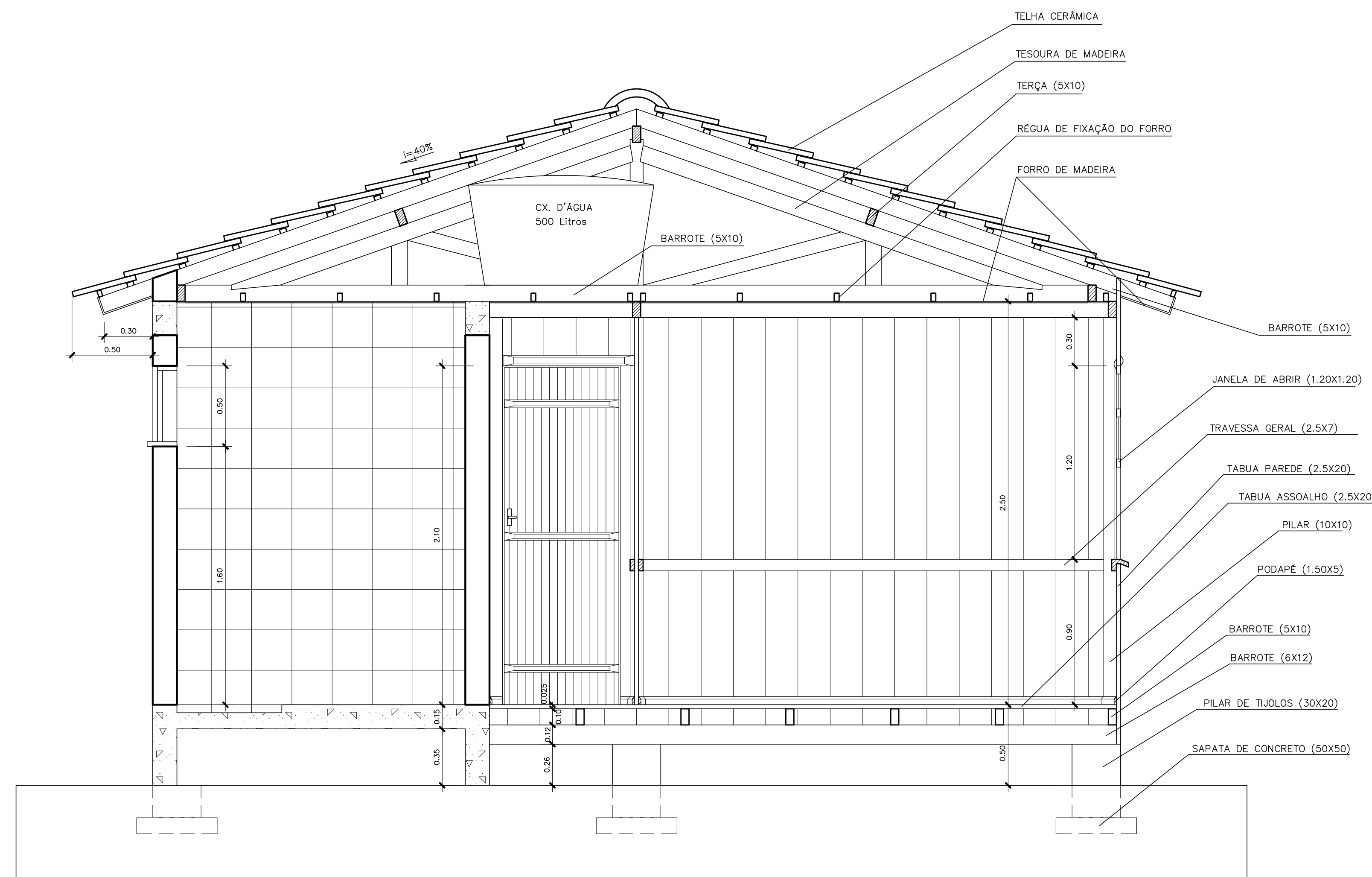
Fachada Escala 1/20
